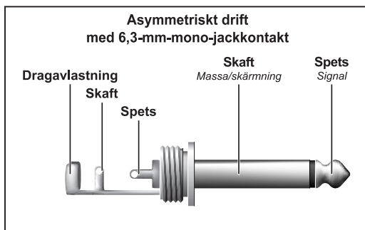
Bild. 5.3: 6,3-mm-Monojackuttag
