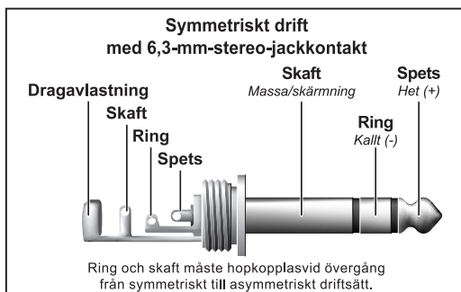
Bild. 5.4: 6,3-mm-Stereojackuttag
