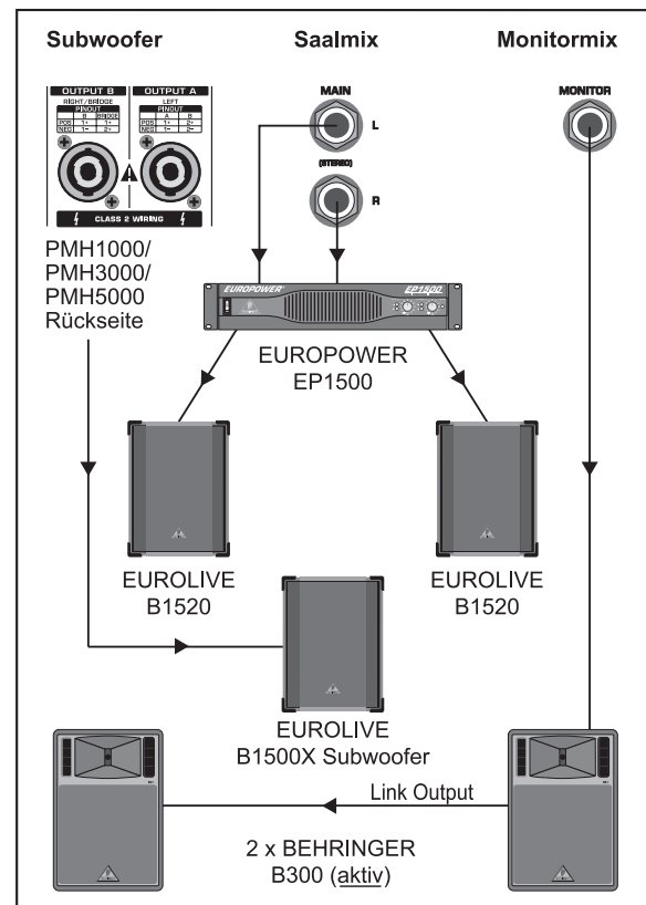
Abb. 5.2: Monobrückenbetrieb
