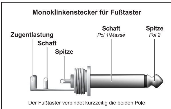
Abb. 4.4: Monoklinkenstecker für Fußtaster
