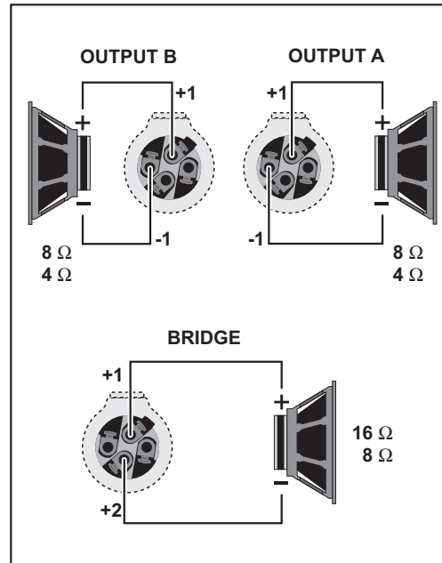
Abb. 4.6: SPEAKON®-Stecker mit Pin-Belegung
