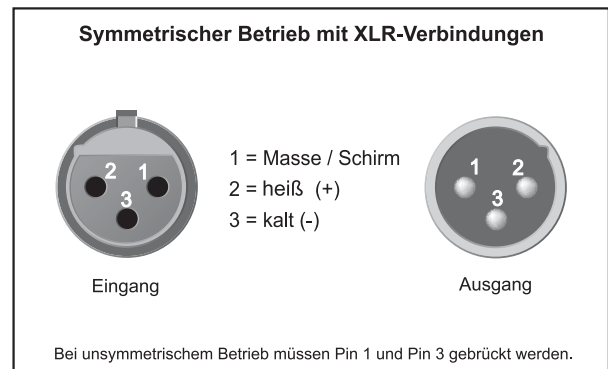
Abb. 4.3: XLR-Verbindungen
