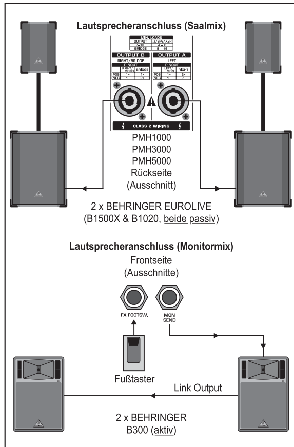
Abb. 5.1: Der EUROPOWER-Mixer als Stereoverstärker
