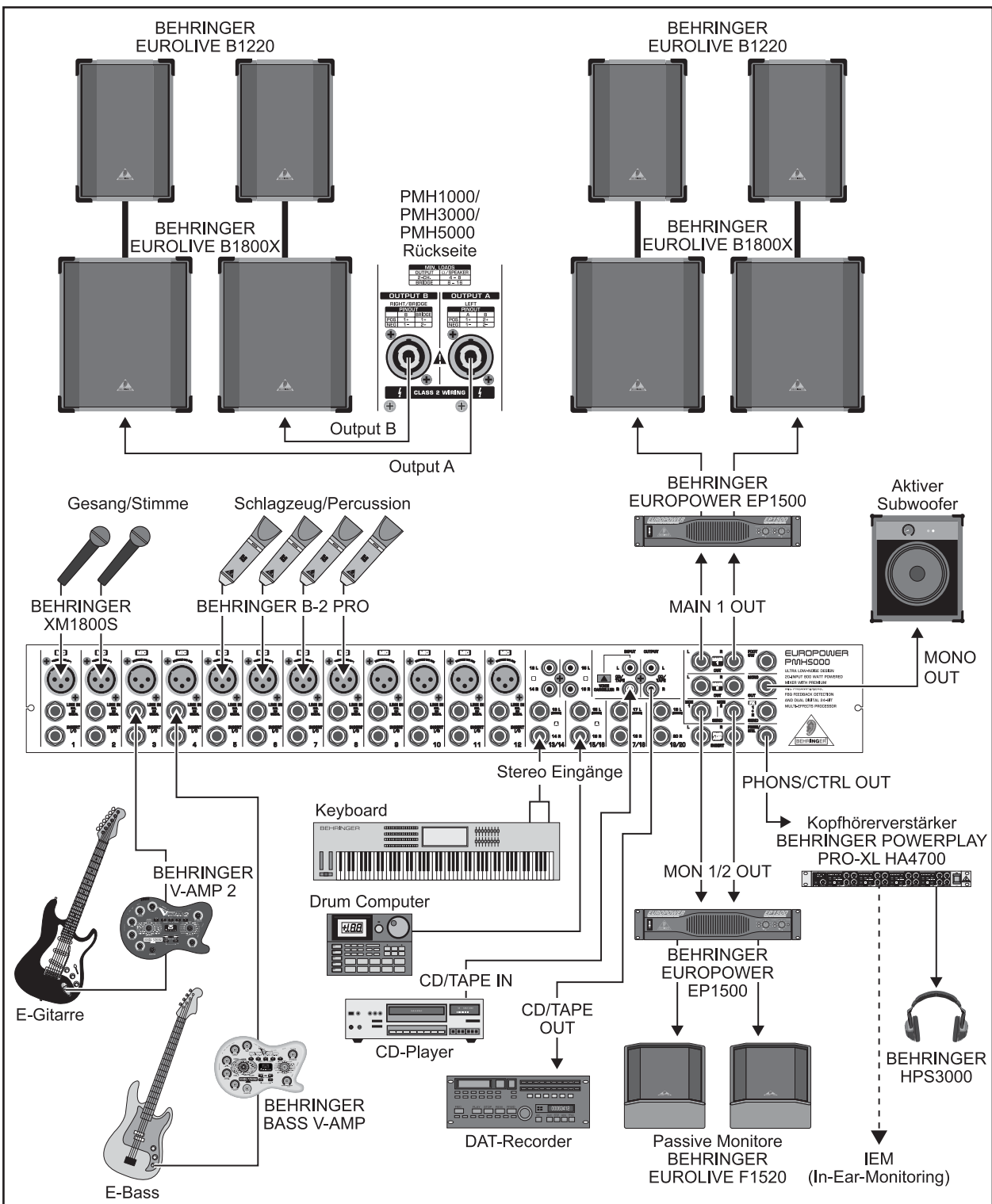
Abb. 5.5: Erweitertes Setup
