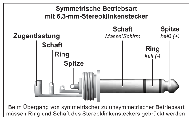
Abb. 4.2: 6,3-mm-Stereoklinkenstecker
