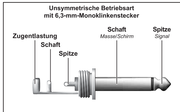
Abb. 4.1: 6,3-mm-Monoklinkenstecker
