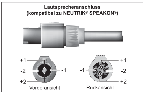
Abb. 4.5: Professioneller Lautsprecheranschluss
