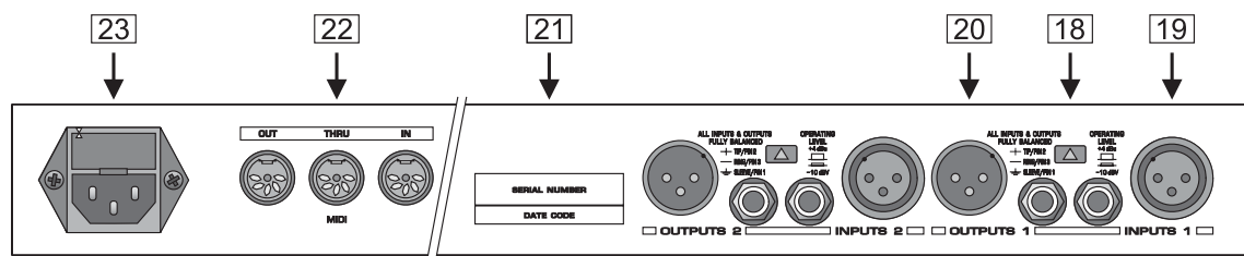
Fig. 1.4 : Les connexions et commandes du panneau arrière
