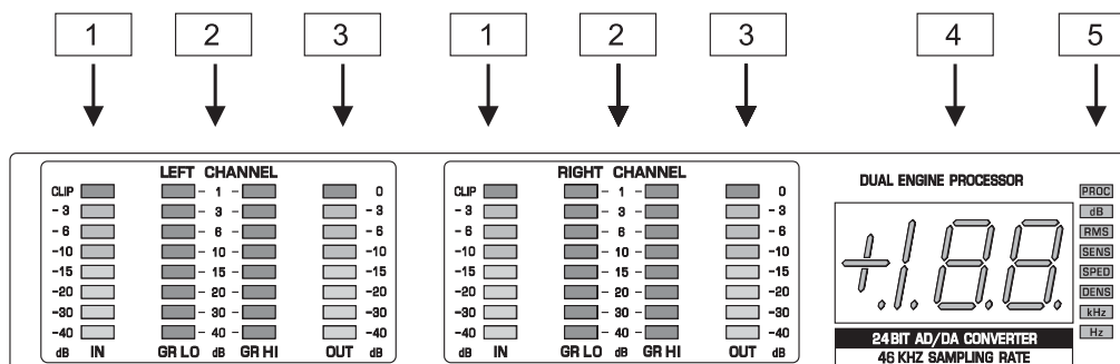
Fig. 1.2 : La section afficheur de l'ULTRAMIZER PRO
