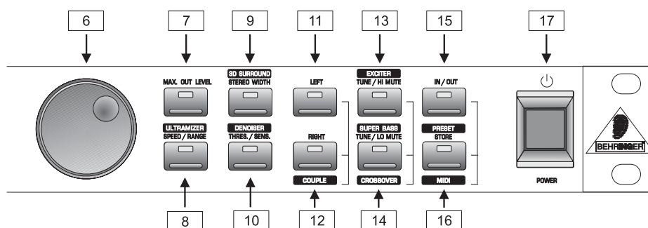
Fig. 1.3 : Les commandes de l'ULTRAMIZER PRO
