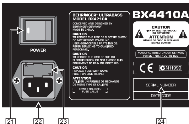
Abb. 2.4: Rückseite des BX4410/BX4410A (Ausschnitt 1)
