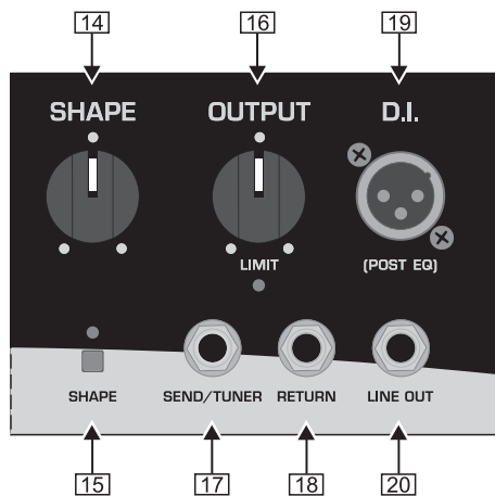
Abb. 2.3: Frontseite des BX4410/BX4410A (Ausschnitt 3)
