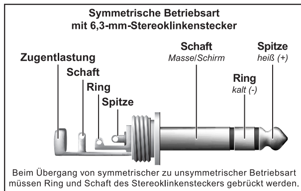
Abb. 6.2: 6,3-mm-Stereoklinkenstecker
