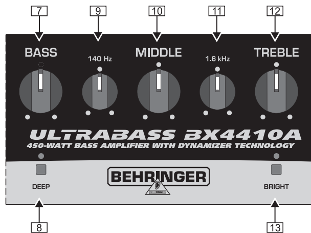
Abb. 2.2: Frontseite des BX4410/BX4410A (Ausschnitt 2)
