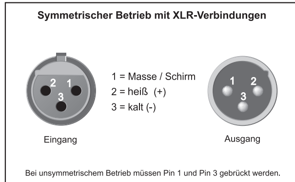
Abb. 6.3: XLR-Verbindungen
