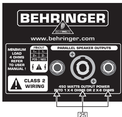
Abb. 2.5: Rückseite des BX4410/BX4410A (Ausschnitt 2)
