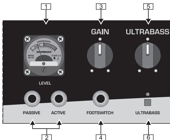
Abb. 2.1: Frontseite des BX4410/BX4410A (Ausschnitt 1)
