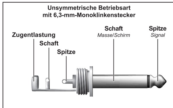
Abb. 6.1: 6,3-mm-Monoklinkenstecker
