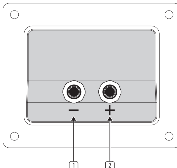
Fig. 2.1: Conectores del panel trasero
