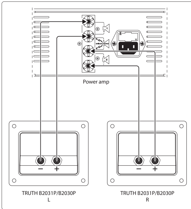
Fig. 3.1: Conexión de un amplificador
